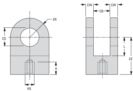
Plain Rod Clevis
